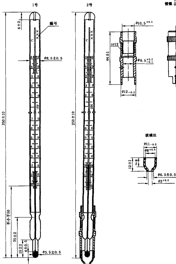
图 5 滴点 1、2 号温度计
