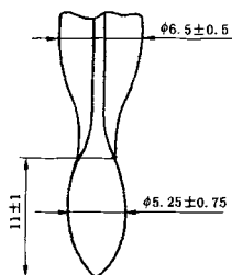
图 18 石蜡冻凝点温度计感温泡示意图
