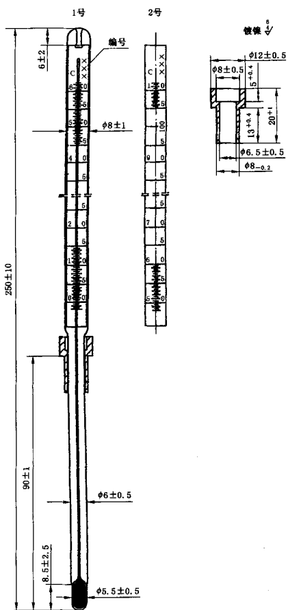
图4 恩氏粘度1、2号温度计
