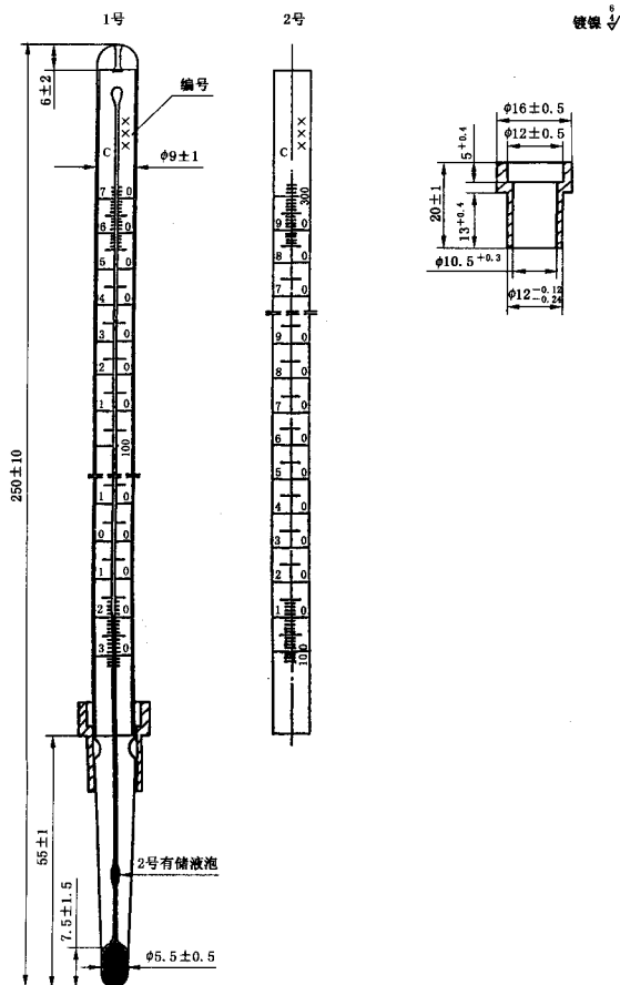
图2 闭口闪点1、2号温度计
