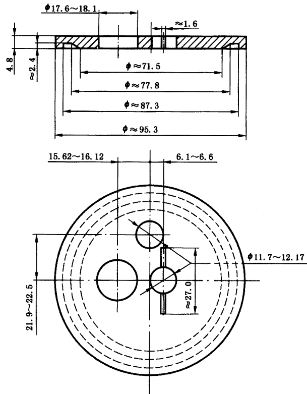
图 2 烧杯盖
