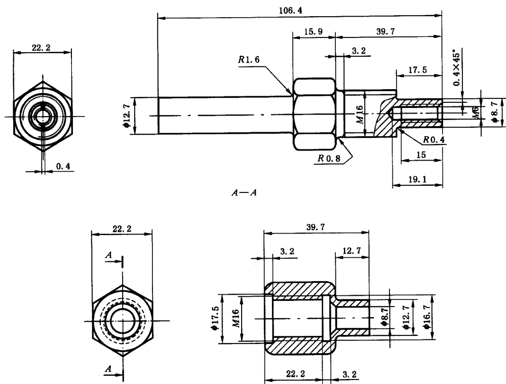
图4 抛光试棒用的夹头
