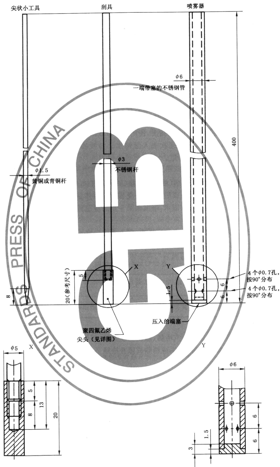
图 2 用于蒸馏仪器的尖状物、刮具、喷雾器
